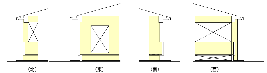
寝室A側ベランダ部分展開図
