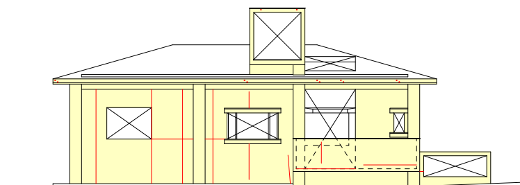
北立面図
