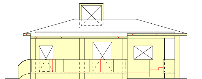
南立面図
