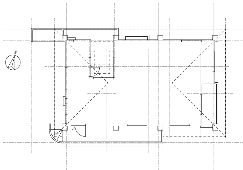
平面図
